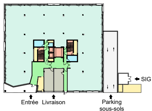
Rez-de-chaussée
