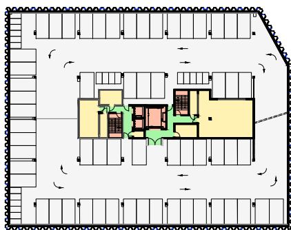
Sous-sol -1
