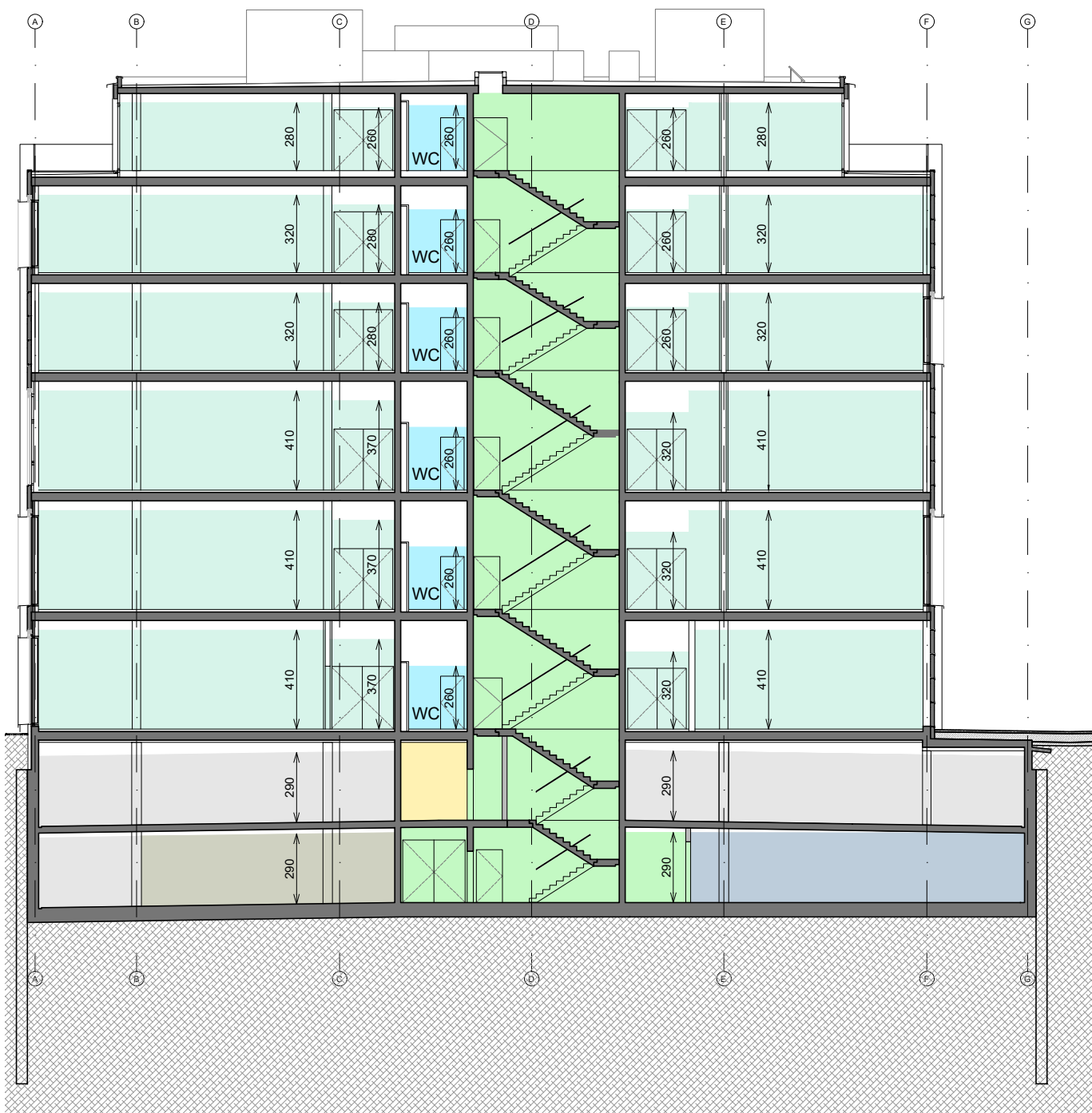
Coupe A-A
